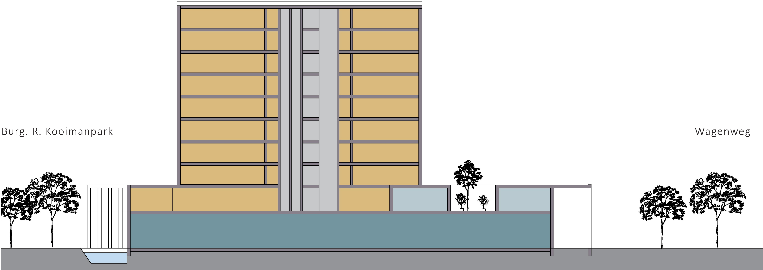
Doorsnede
